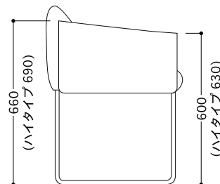
[アーム高さ]
